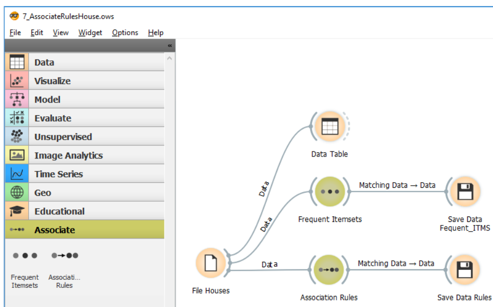
Obr. 124 Workflow pro frekventované sady a asociační pravidla
