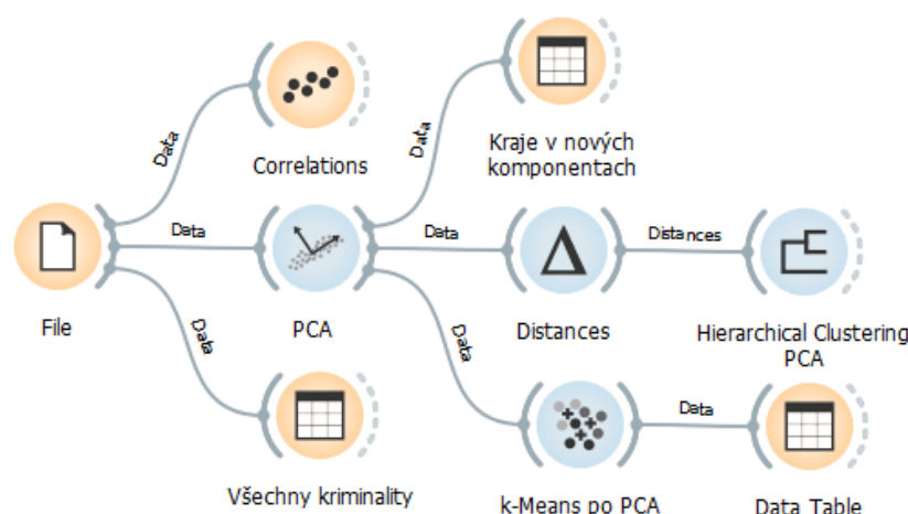
Obr. 77 Hierarchické shlukování krajů podle druhů kriminálních činů po transformaci pomocí PCA
