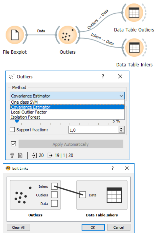
Obr. 13 Workflow s uzlem Outliers a nastavení spojných čar v dialogu Edit Links pro specifikaci výstupu
