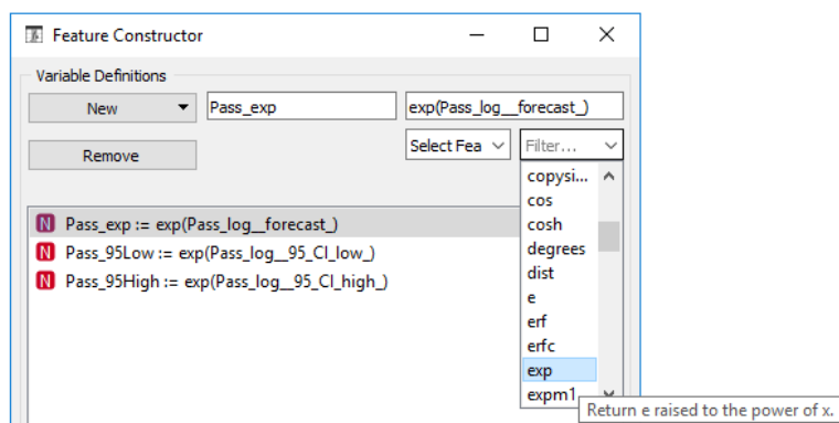
Obr. 196 Přepočet predikovaných hodnot do původních jednotek exponenciální funkcí
