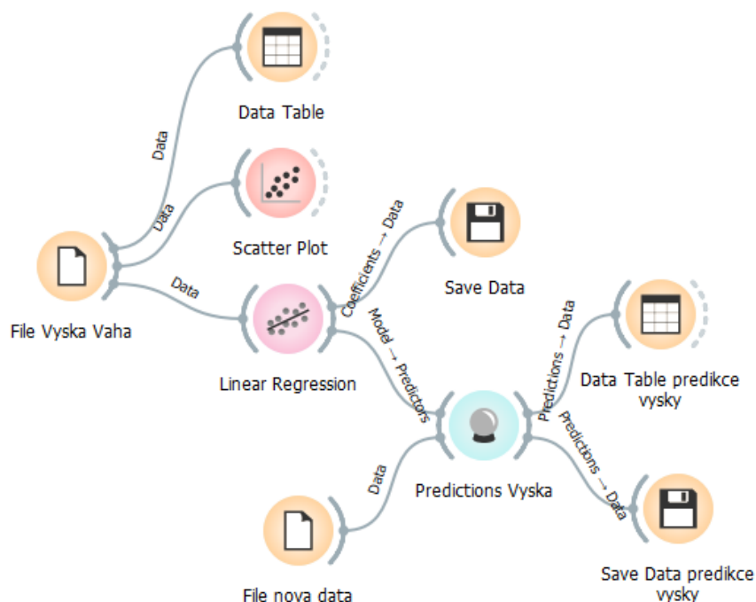
Obr. 89 Workflow predikce hmotnosti pomocí lineární regrese
