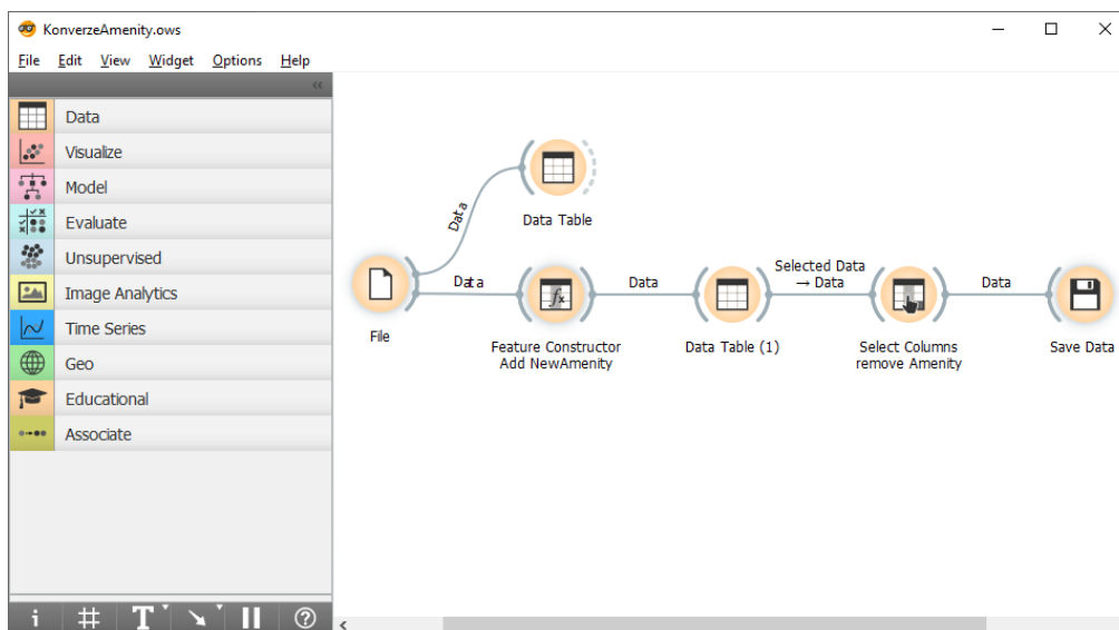
Obr. 3 Základní rozhraní software Orange
