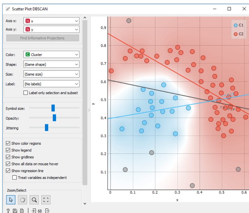
Obr. 86 Výsledek shlukování metodou DBSCAN
