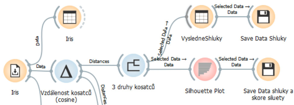
Obr. 63 Workflow s uzlem Silhouette Plot pro posouzení výsledku shlukování
