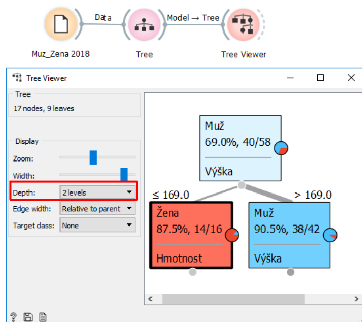
Obr. 102 Rozhodovací strom do druhé úrovně větvení
