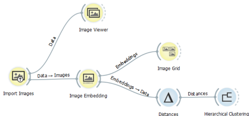
Obr. 140 Workflow pro hierarchické shlukování obrázků na základě klasifikace pomocí natrénované neuronové sítě v uzlu Image Embedding
