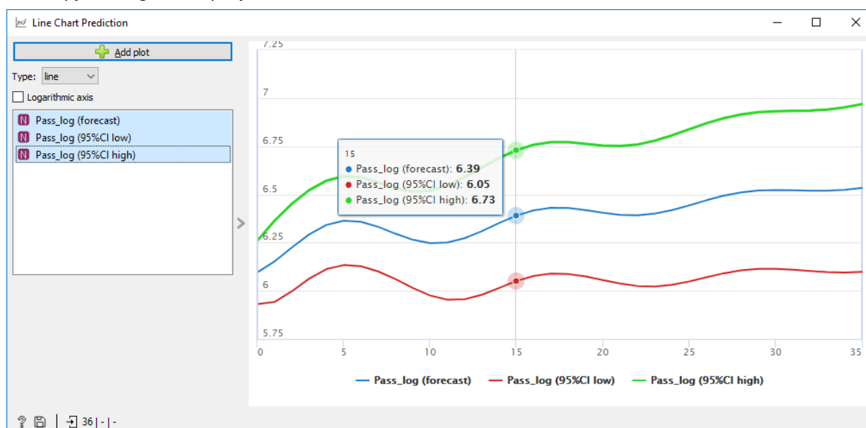
Obr. 194 Predikce na následující tři roky v logaritmických hodnotách
