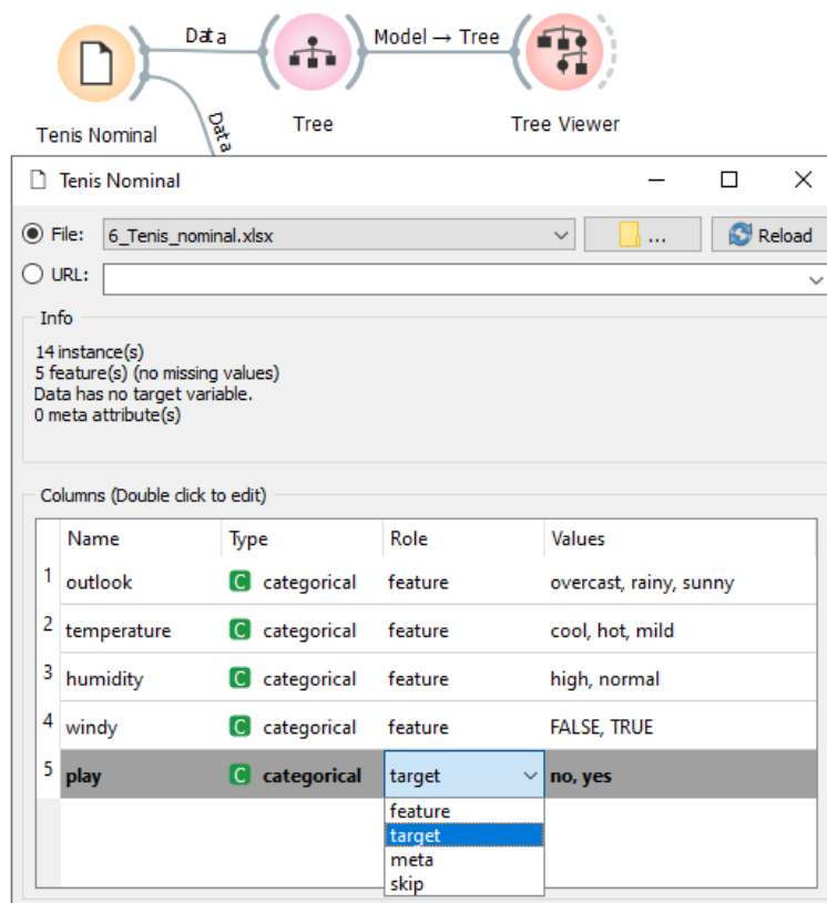
Obr. 97 Workflow a nastavení vstupních dat
