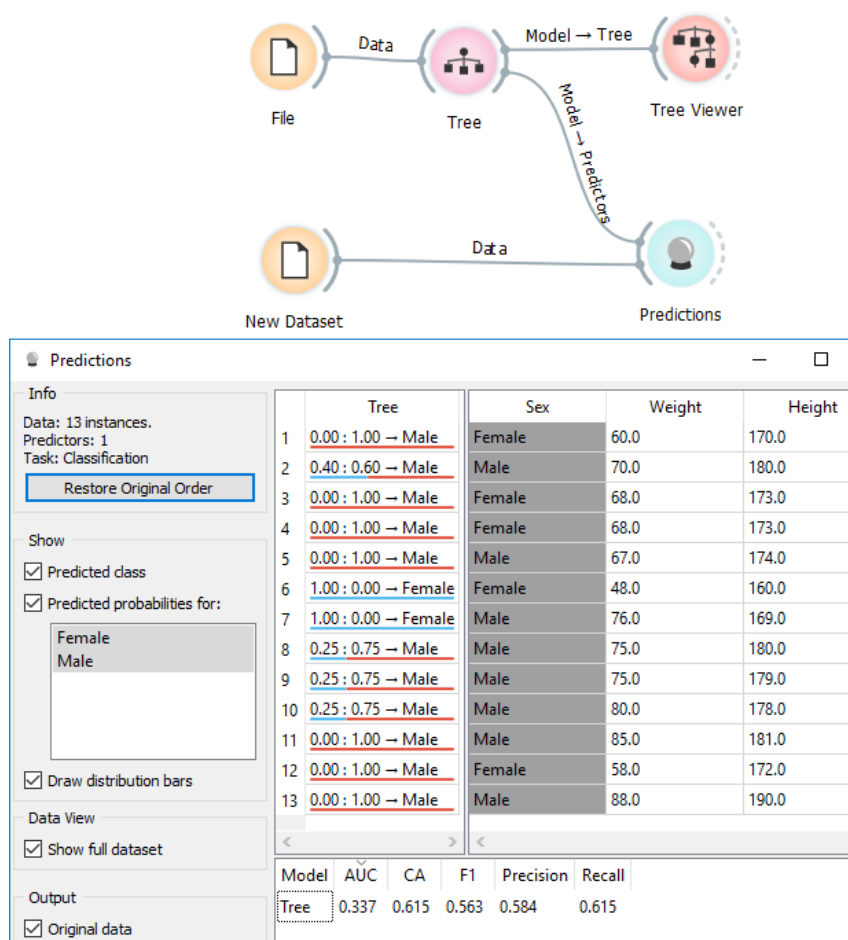
Obr. 104 Výsledek predikce pohlaví
