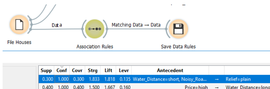
Obr. 131 Výběr asociačního pravidla pro uložení odpovídajících instancí
