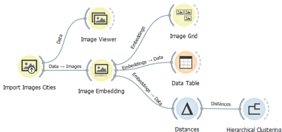
Obr. 153 Workflow pro nalezení podobných měst podle landuse
