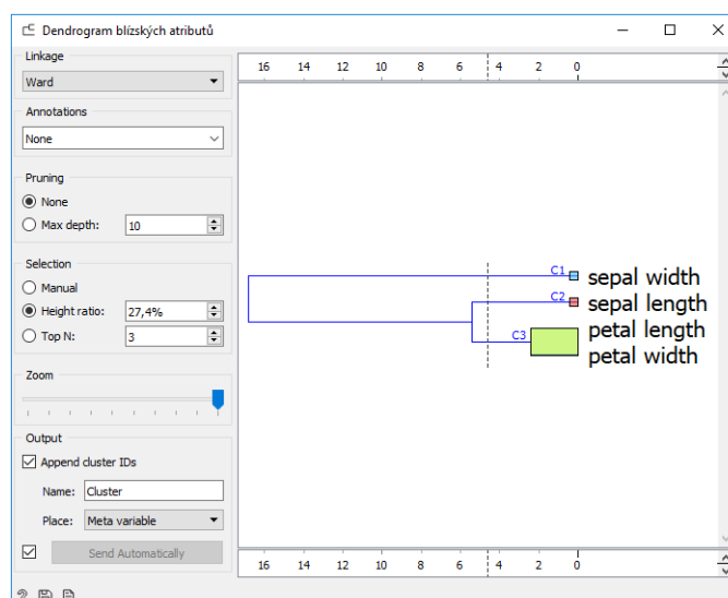
Obr. 66 Výsledný dendrogram podle hodnot atributů květních lístků
