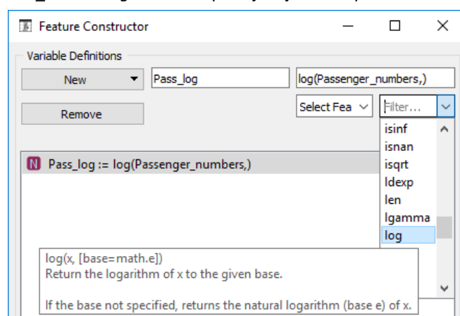
Obr. 192 Logaritmování vstupních hodnot
