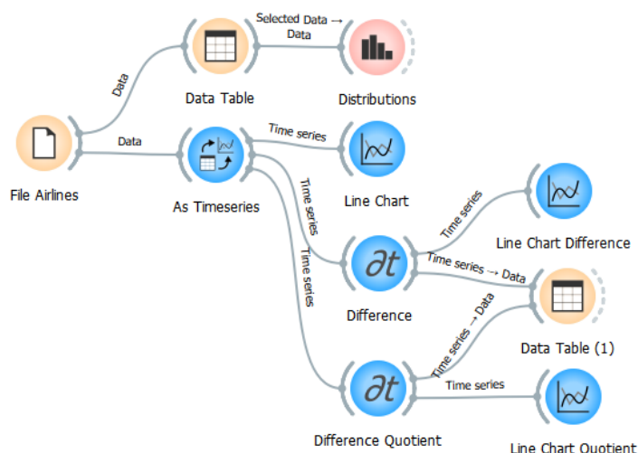
Obr. 178 Workflow pro časovou řadu počtu pasažérů
