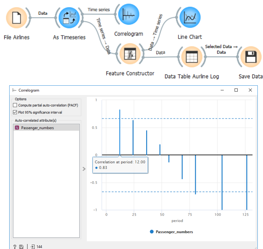
Obr. 191 Workflow a korelogram – graf autokorelační funkce
