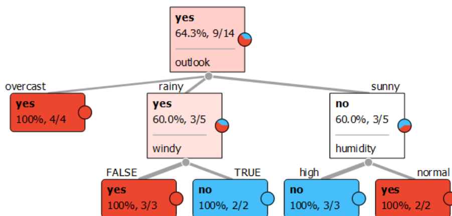
Obr. 98 Výsledný strom
