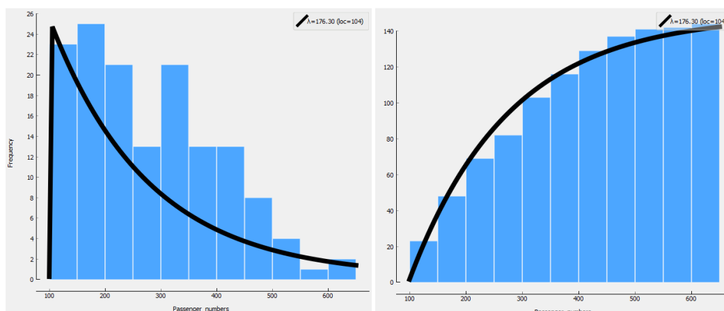
Obr. 180 Histogram hodnot počtu pasažérů za celé časové období (a), kumulativní distribuce (b)
