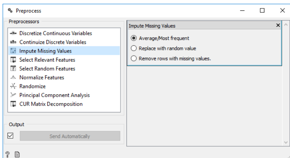
Obr. 26 Možnosti imputace chybějících hodnot pomocí uzlu Preprocess
