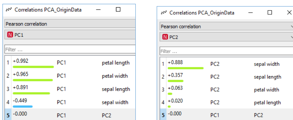
Obr. 44 Korelace původních atributů a nových komponent PC1 (vlevo) a PC2 (vpravo)
