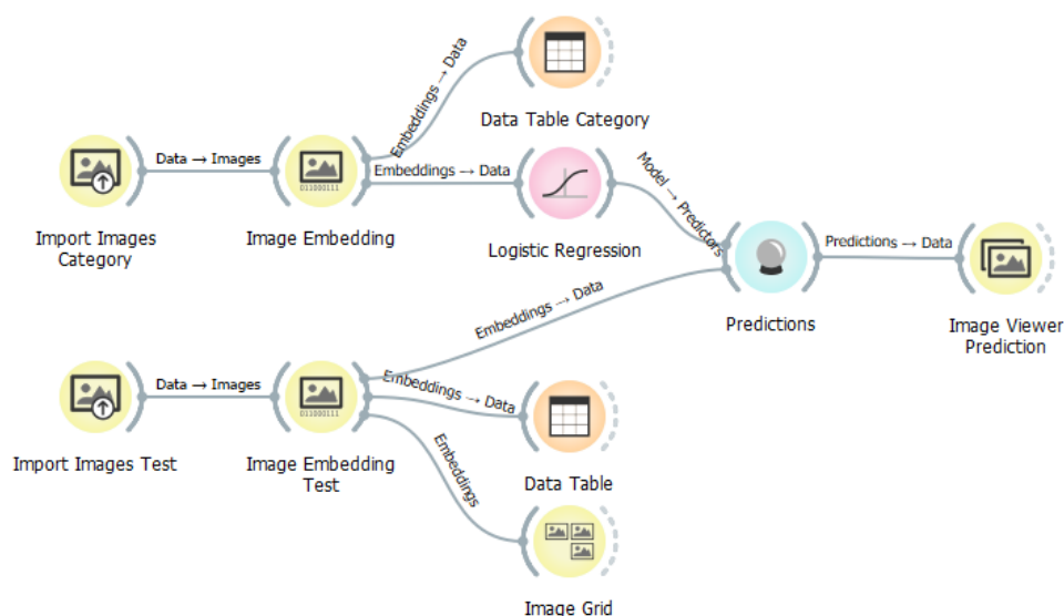
Obr. 151 Workflow pro určení druhu mapy na základě testovacích dat
