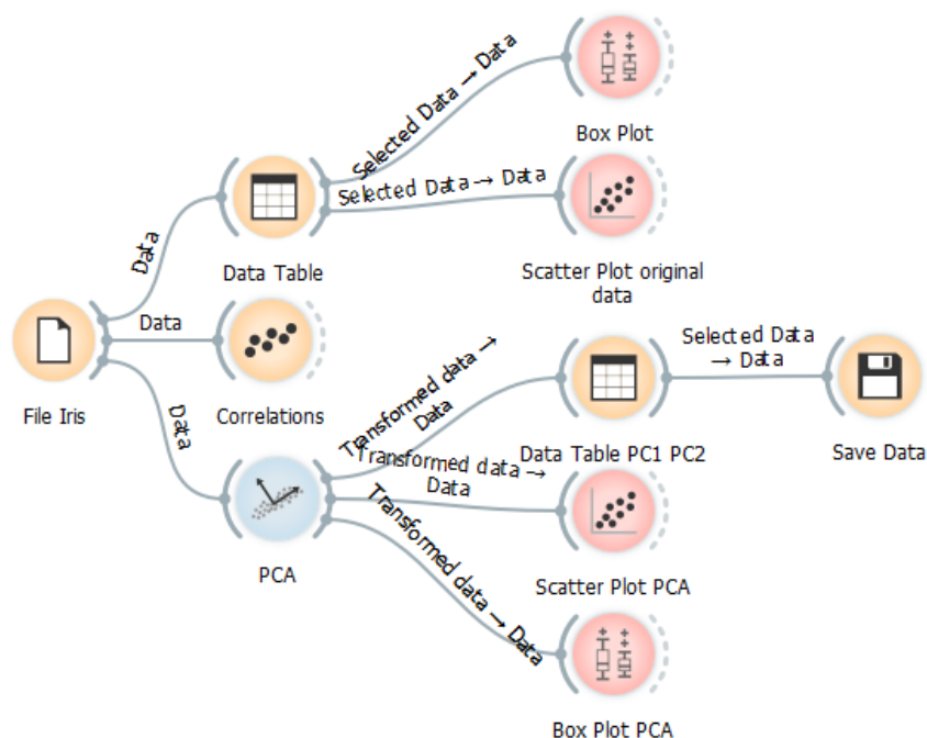
Obr. 37 Workflow s transformací pomocí metody PCA
