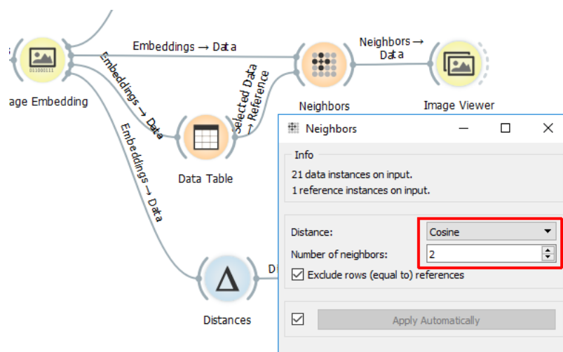
Obr. 147 Nastavení uzlu Neighbors pro hledání podobných map
