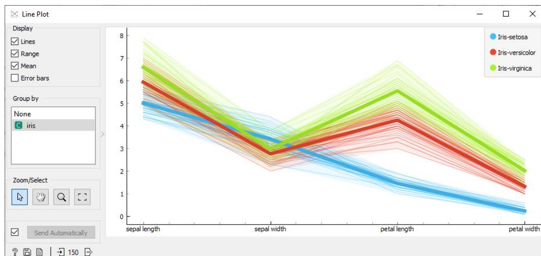
Obr. 17 Paralelní graf čtyř atributů datasetu Iris
