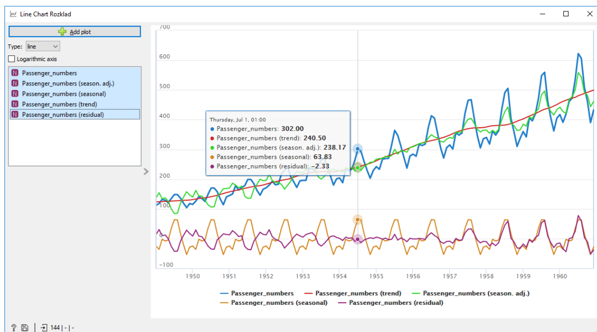
Obr. 189 Aditivní rozklad řady nestacionární řady
