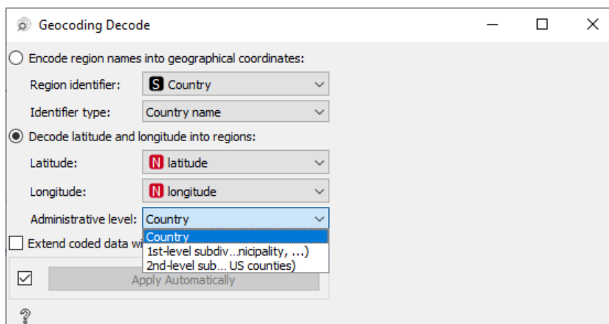
Obr. 165 Nastavení dekódování
