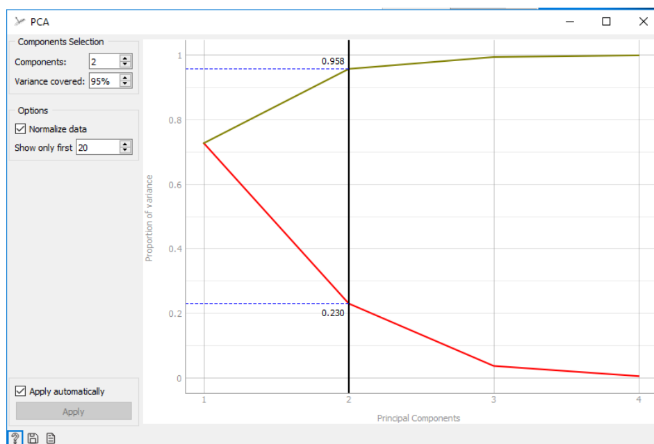
Obr. 38 Sutinový graf vlastních čísel (scree plot)
