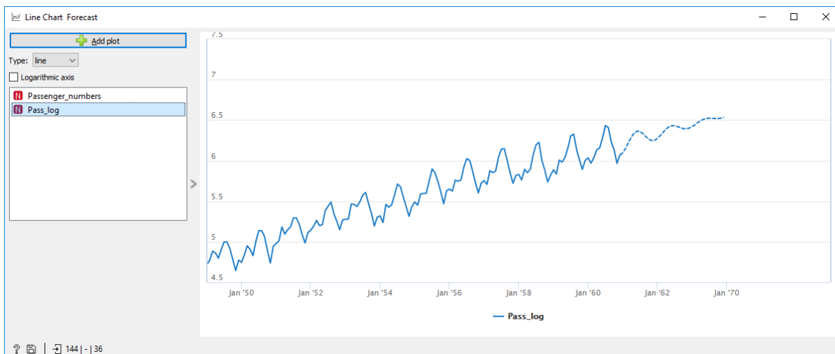
Obr. 195 Zobrazení původní časové řady a predikce ARIMA modelem v logaretmických jednotkách
