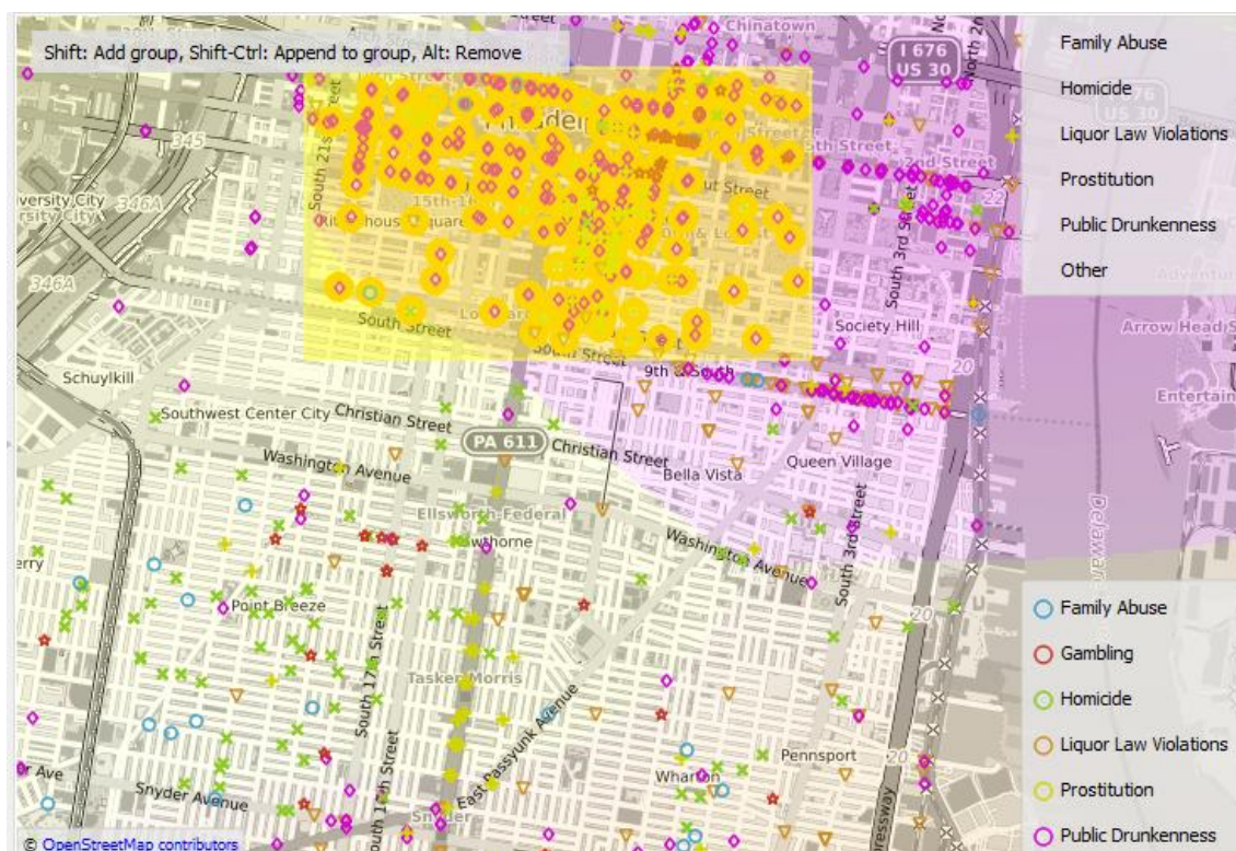
Obr. 160 Výběr obdélníkové oblasti pro následnou možnost uložení výběru dat do tabulky. Fialově je vykreslena oblast, kde převládá Public Drunkenness (zapnuta volba Show color region)
