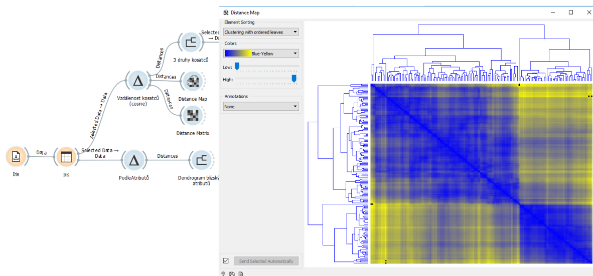
Obr. 67 Matice vzdáleností zobrazená pomocí uzlu Distance Map
