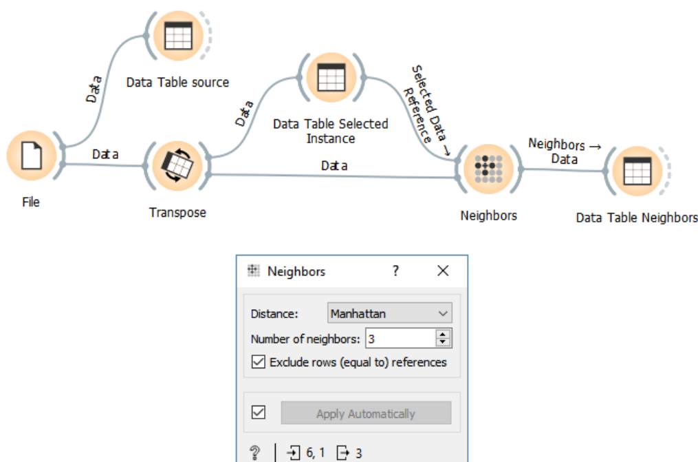
Obr. 79 Workflow s uzlem Neighbors pro zjištění nejbližších instancí
