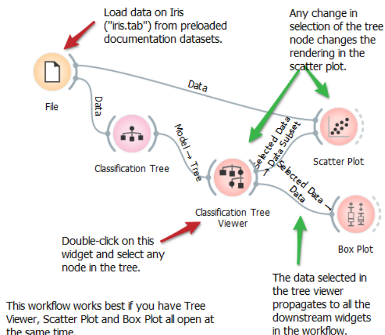
Obr. 94 Ukázkové workflow dodávané s Orange včetně komentářů
