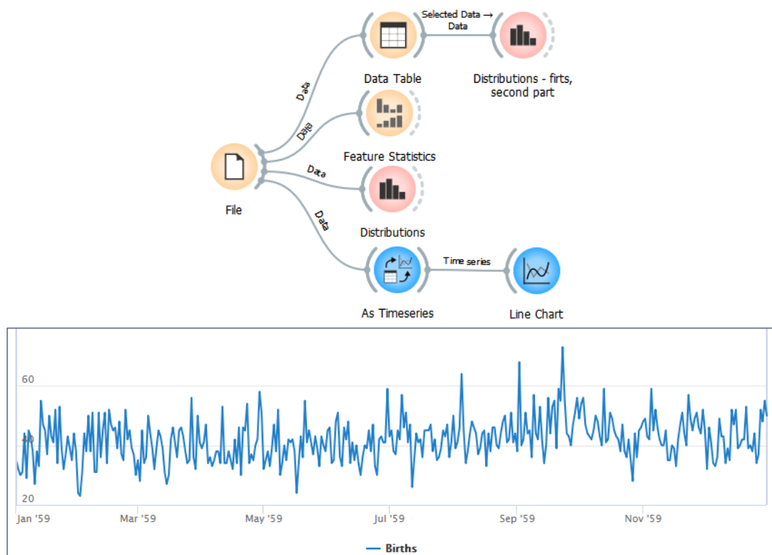
Obr. 174 Workflow a časová řada počtu narozených žen v průběhu jednoho roku zobrazená uzlem Line Chart
