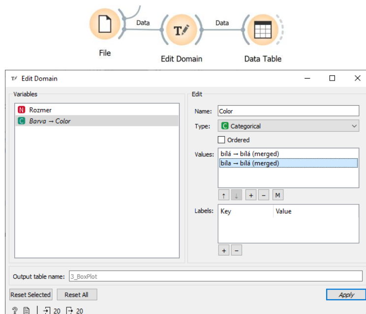
Obr. 22 Nastavení editace hodnot domény pomocí uzlu Edit Domain
