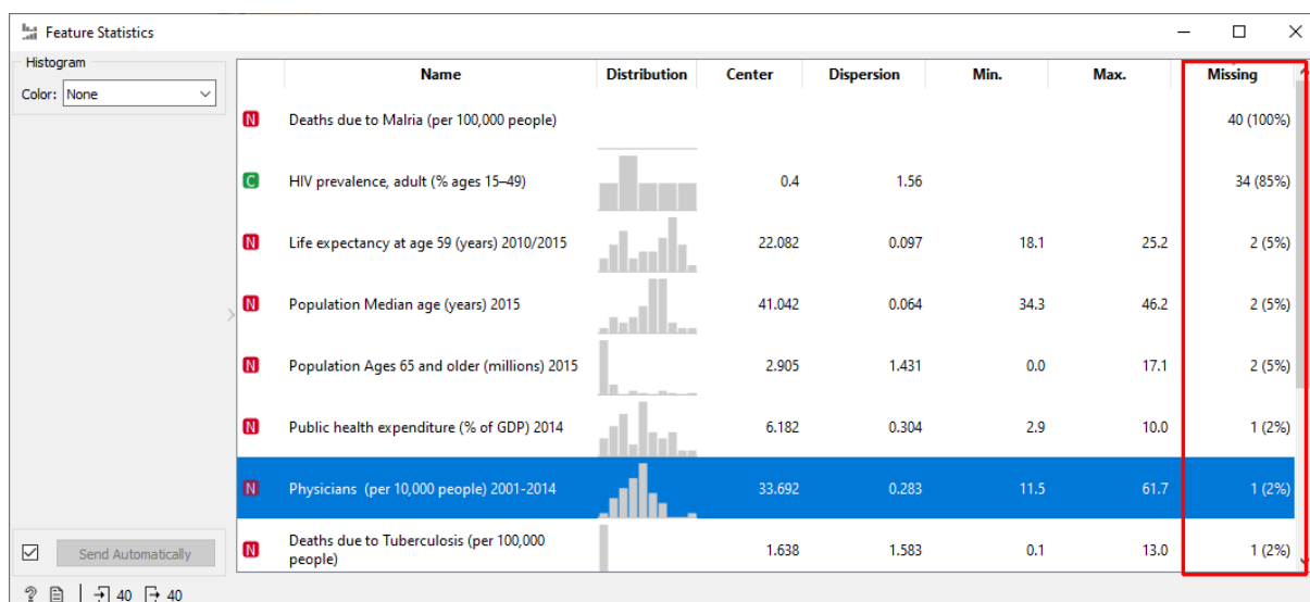
Obr. 24 Zjištění chybějících hodnot pomocí uzlu Feature Statistics
